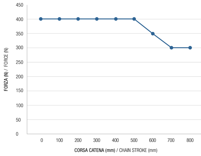
L40 Slim - 800 - Portate attuatori vasistas L40 Slim - 800 - Actuator force - bottom hung
