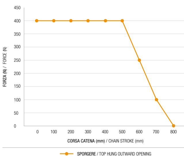
L40 Slim - 800 - Portate attuatori a sporgere L40 Slim - 800 - Actuator force - top hung and dome
