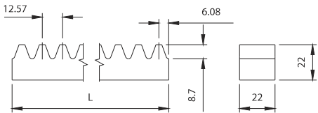
Modulo m=4
