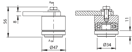
SEZ. A-A
